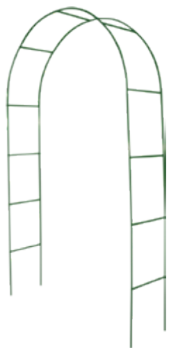
АРКА САДОВАЯ ДЛЯ ВЬЮЩИХСЯ РАСТЕНИЙ НФО014 Длина 370 мм Ширина 1400 мм Высота 2400 мм
