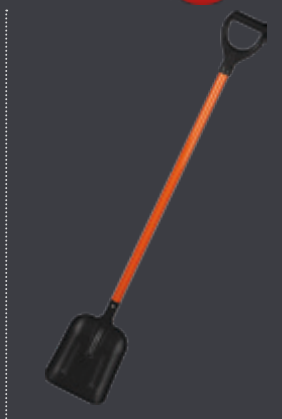
ЛОПАТА СОВКОВАЯ "ЛЮКС" Материал: сталь 3 (толщина 1,5 мм), пластмасса. Сварная тулейка Размер: 1500x235x60 мм.
