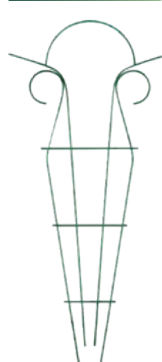
ШПАЛЕРА "ТЮЛЬПАН" Ширина 720 мм Высота 1900 мм
