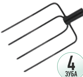
ВИЛЫ НАВОЗНЫЕ (А) СВАРНЫЕ Сварные. Размер: 38x22 см. Материал: сталь. Профиль 8 мм. Диаметр тулейки 36 мм.
